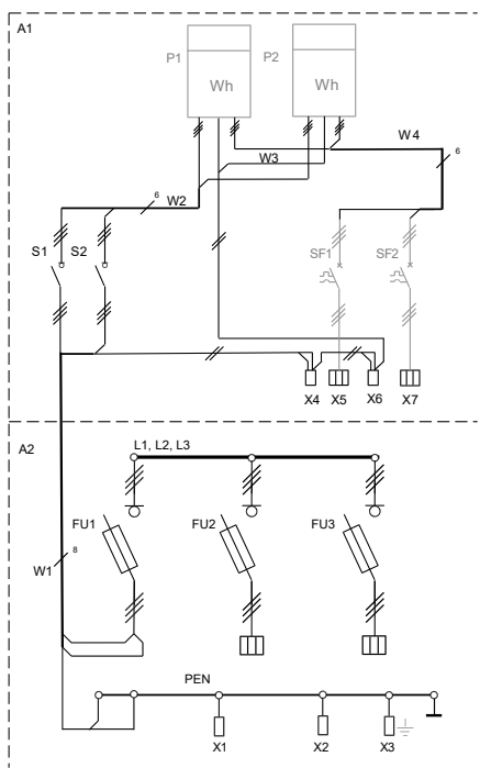
1. att. Elektriskā principshēma
