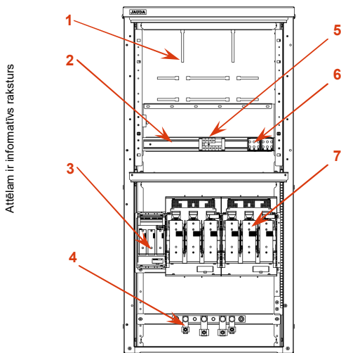
2. att. Aparatūras un elementu izvietojums
